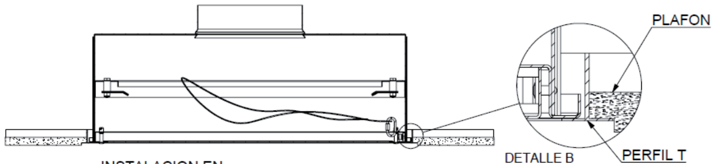
INSTALACION EN PLAFON RETICULAR
