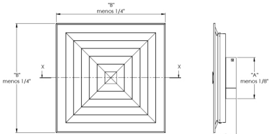
Apertura de Plafón Tamaño de Plato "B" menos 1/2"
