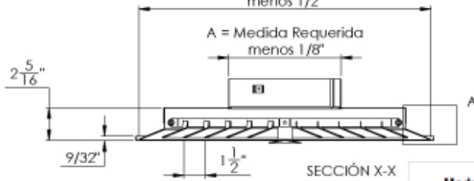
SECCIÓN X-X
