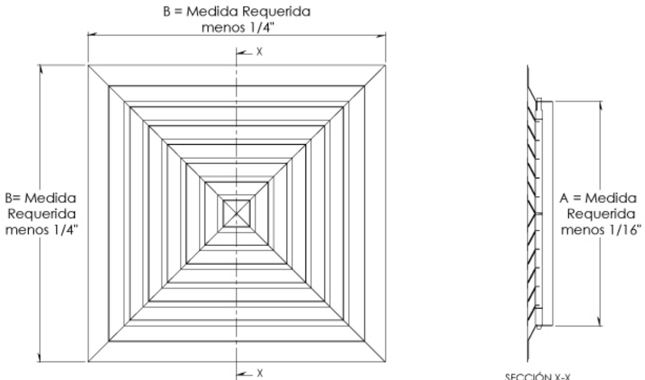
SECCIÓN X-X
