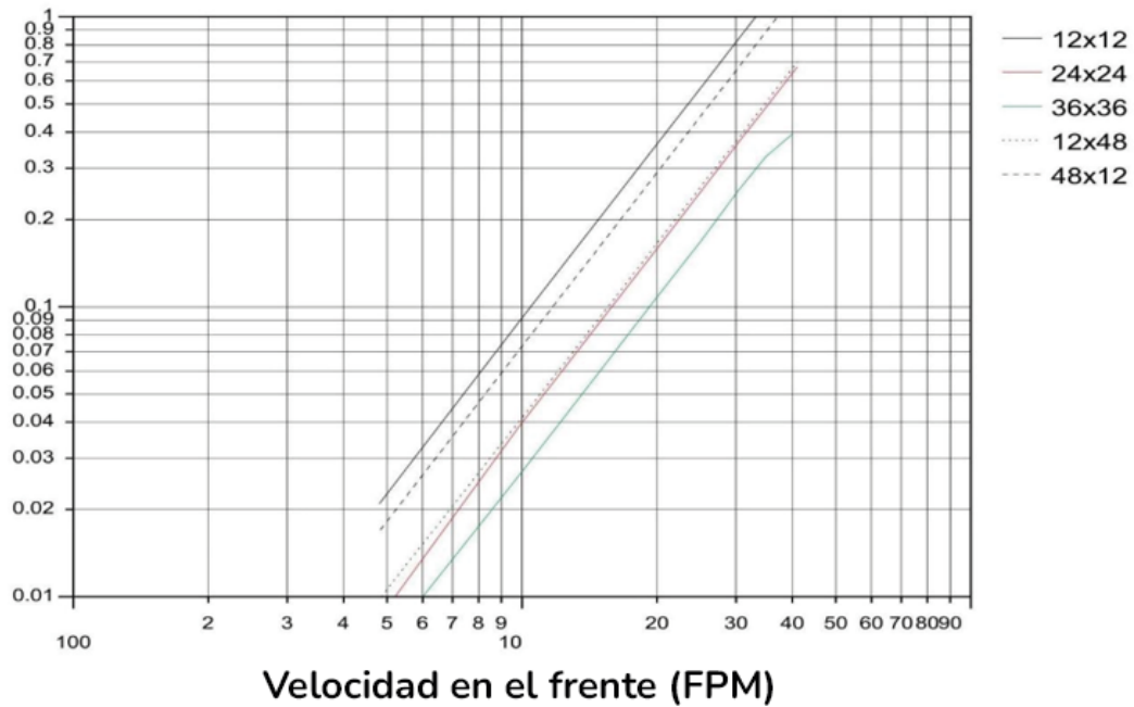
Velocidad Vs Caída de Presión
