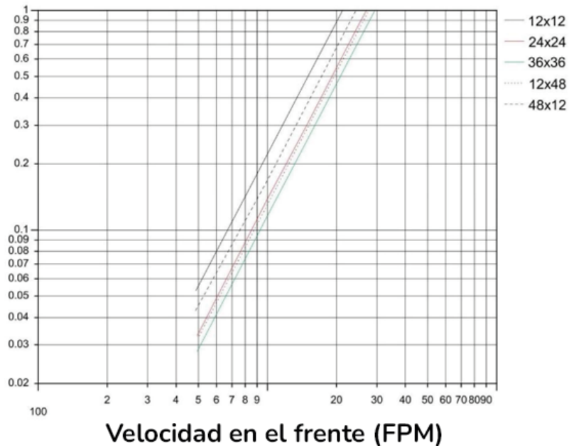
Velocidad Vs Caída de Presión
