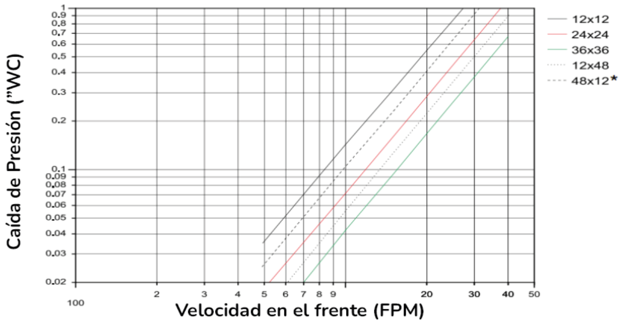
Velocidad Vs Caída de Presión
