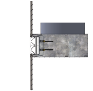
DIFUSOR INSTALADO EN PLENUM MEDIANTE PUENTE
