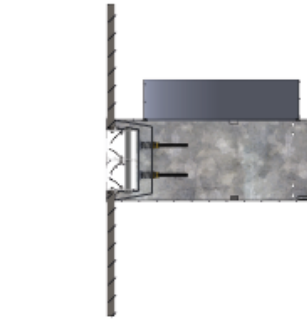
DIFUSOR INSTALADO EN PLENUM MEDIANTE PUENTE
