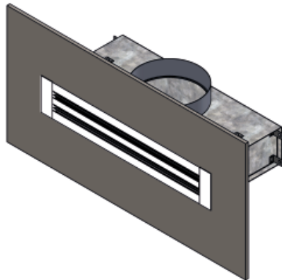
Modelo CAP: Montaje con puente opcional
