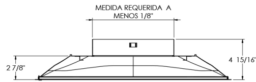
SECCIÓN X-X
