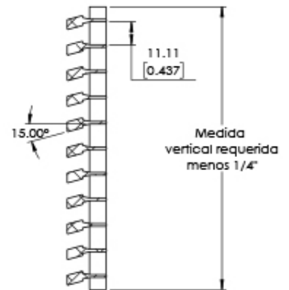
SECCIÓN X-X
