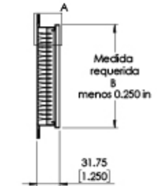
SECCIÓN Y-Y
