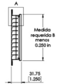
SECCIÓN Y-Y
